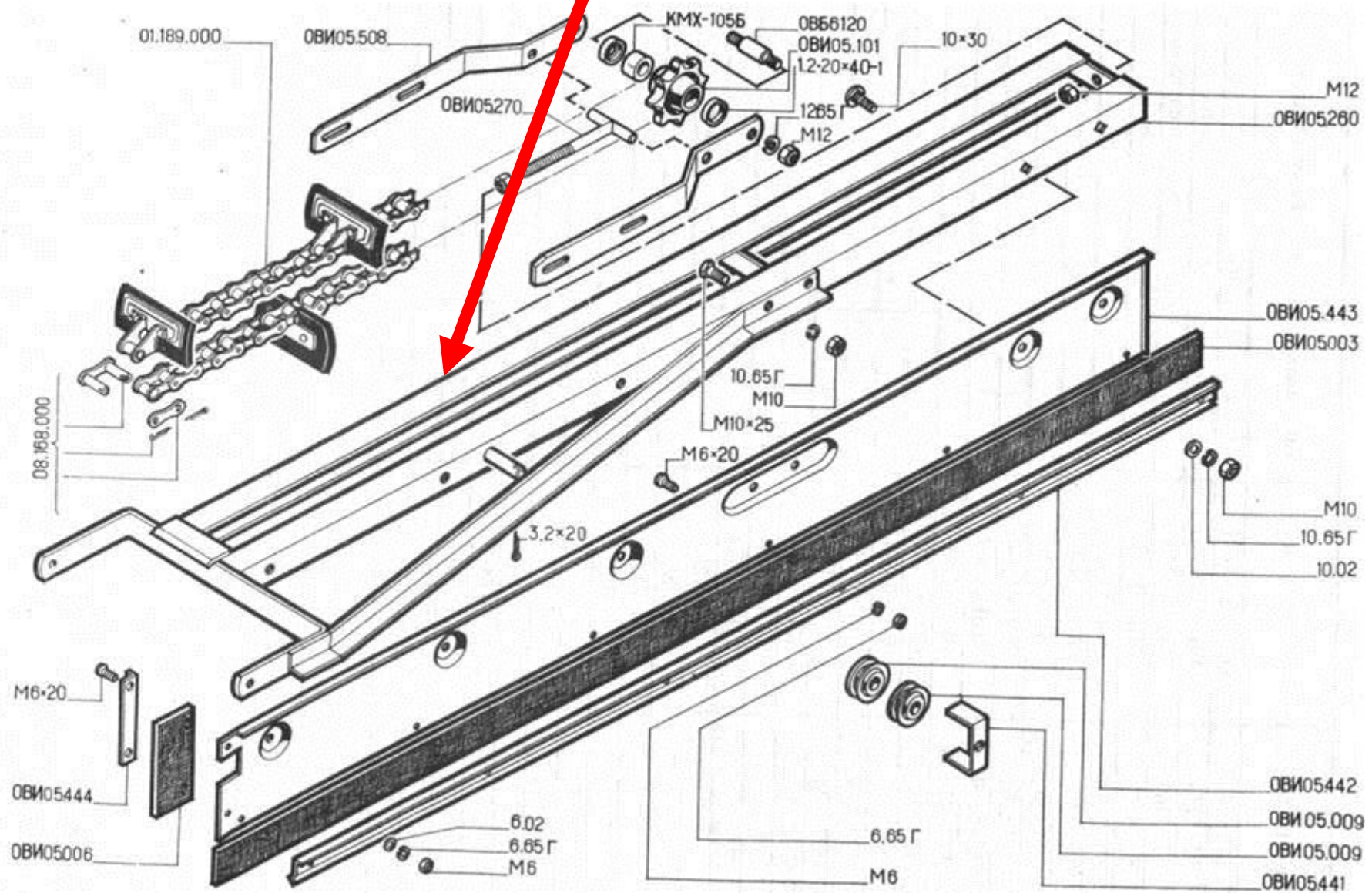
Рис. 26. Питатель ОВИ 05.200.
